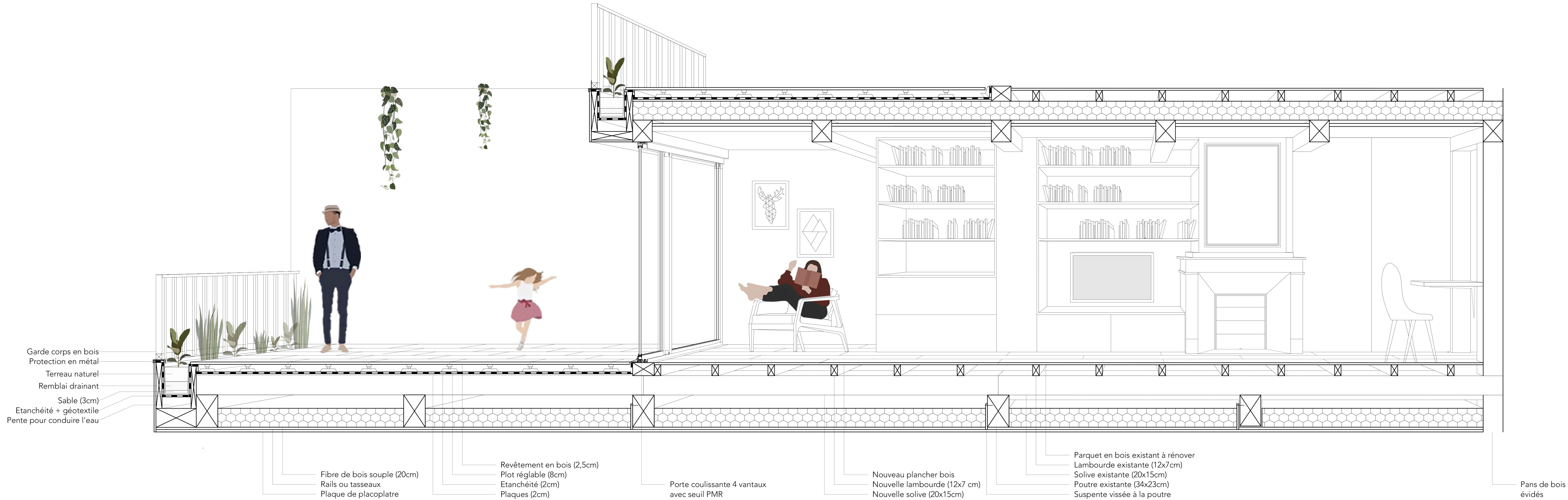
Coupe perspective
